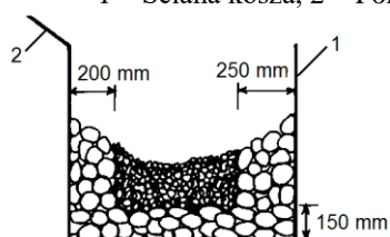
Rys. 4. Wypełnienie kosza gabionowego dwoma rodzajami materiałów; z zewnątrz – kamień grubo, w środku – piasek, kamienie drobne, gruz betonowy itp.
